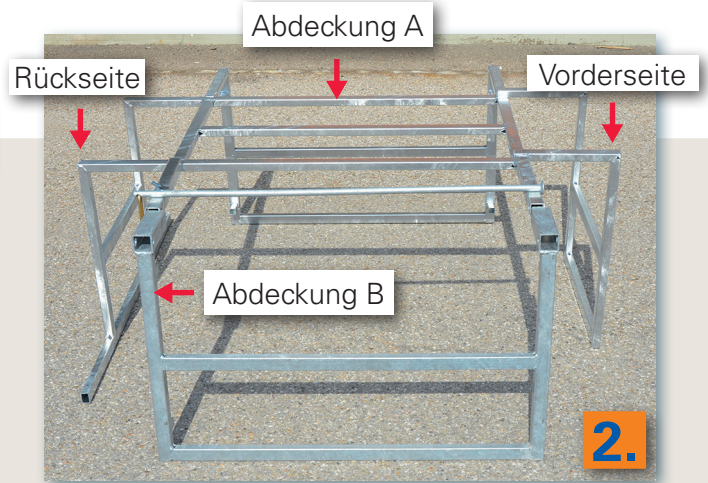
Vier Komponenten sichern die Palette: Abdeckung A, Abdeckung B, Sicherungsstange, Schloss.
